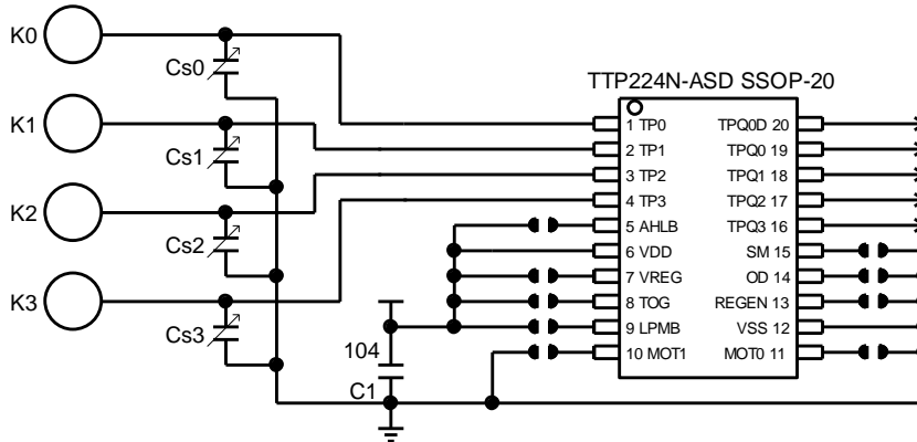
TTP224N-ASD APPLICATION (enable internal regulator)
