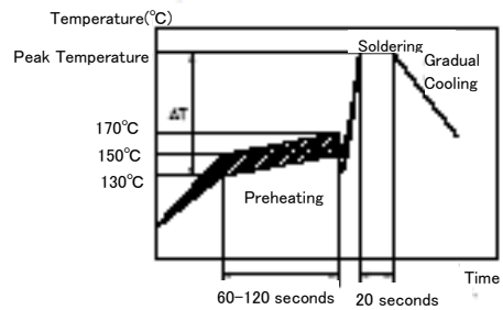
Vapor Reflow
