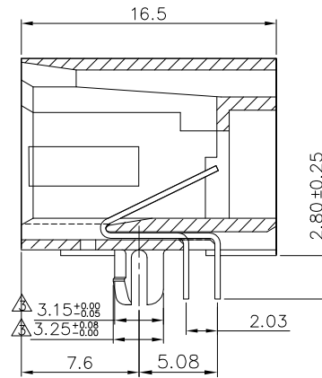
SECCION E-E
