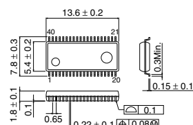
SSOP-B40
