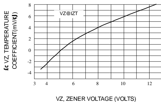
Fig. 2-ZENER VOLTAGE-TO 12 VOLTS
