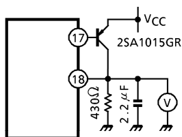
(10) V_{REG}
