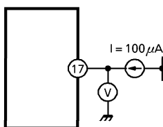
(11) V_{REG L}
