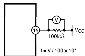
(12) V_{RSSI}
