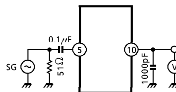
(12) V_{RSSI}
