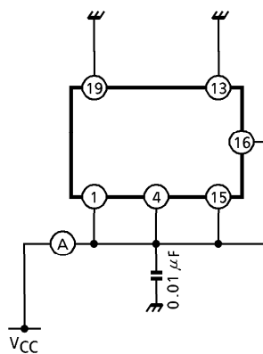
I_{CCO}
