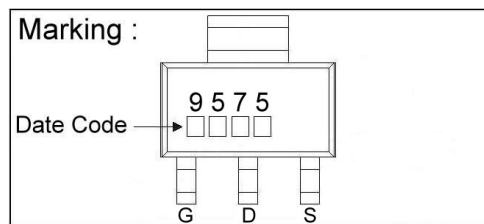
SOT-223
