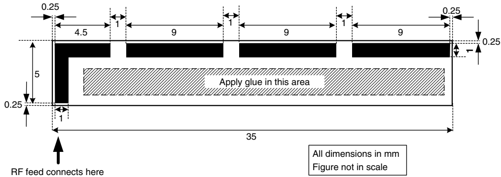
Fig. 4 - VJ 3505 Footprint
