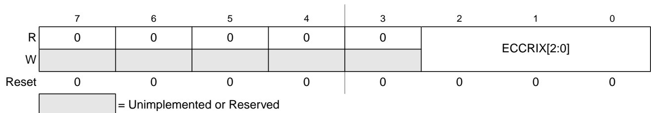
Figure 7-8. FECCR Index Register (FECCRIX)
