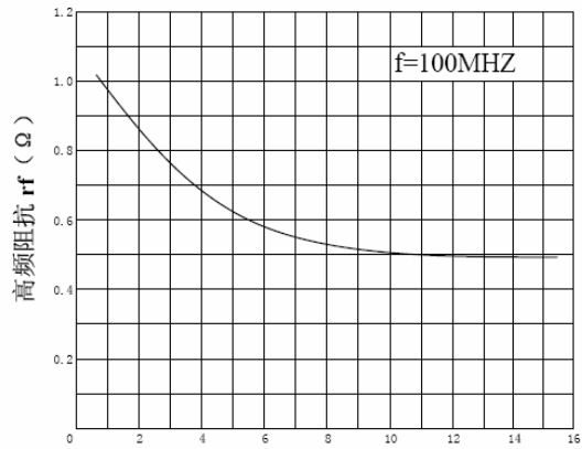
正向电流 I_F (mA)
