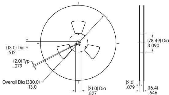
Reel Dimensions
