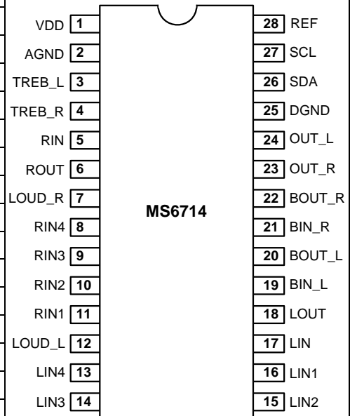
SOP28 / SSOP28
