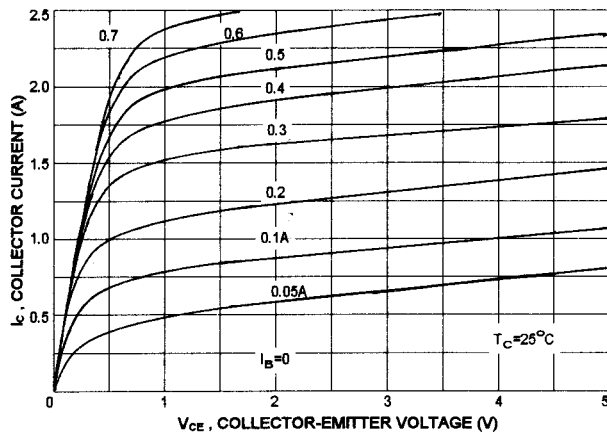
IC - Vce
