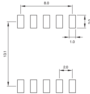
LAND PATTERNS(mm) 推奨ランド寸法
