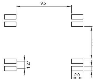
LAND PATTERNS(mm) 推奨ランド寸法
