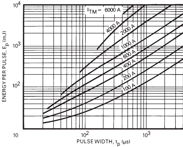
FIG.12 ENERGY PER PER FOR TRAPEZOIDAL PULSES
