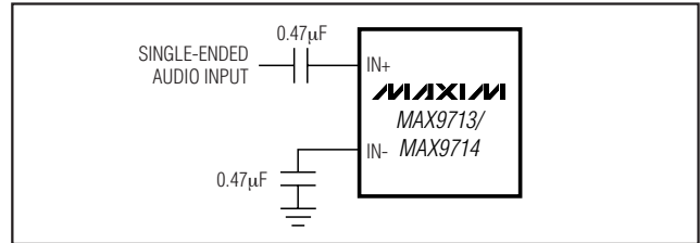
图5. 单端输入
