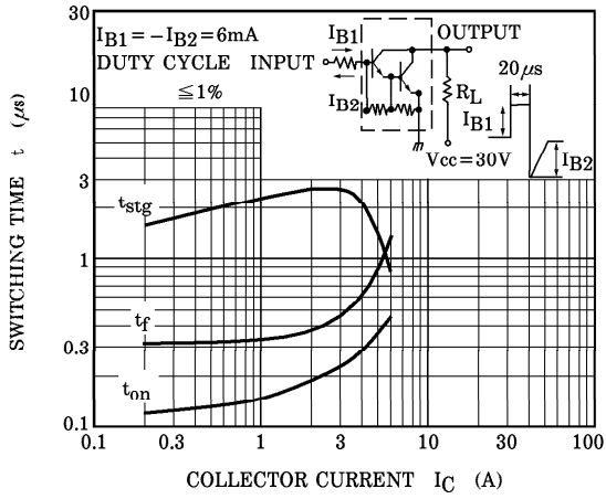
スイッチング特性 (NPN)
