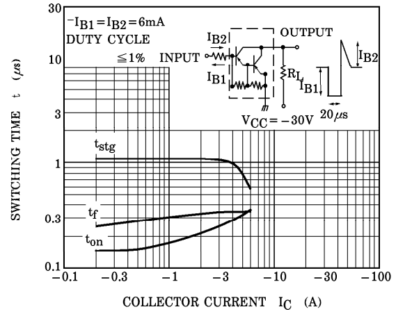
スイッチング特性 (PNP)
